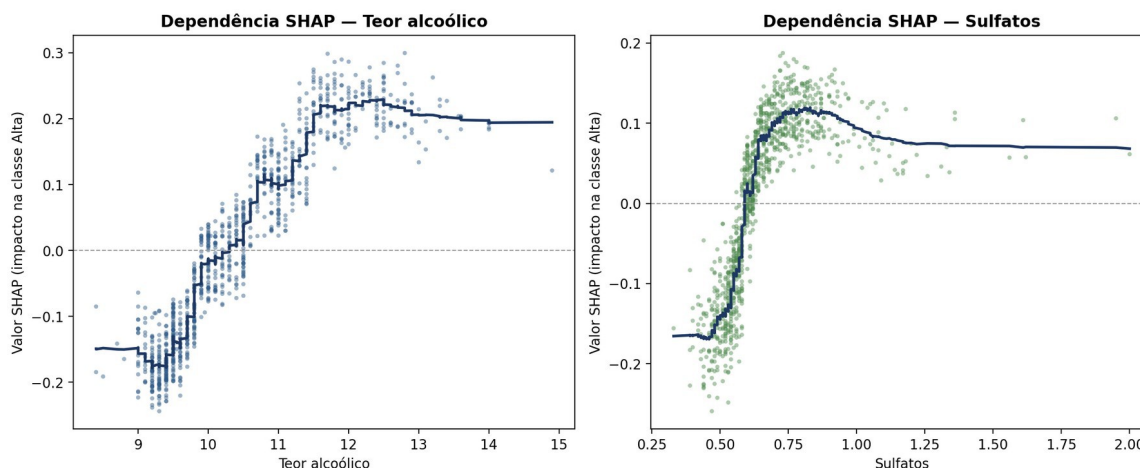
Figura 17 — Dependência SHAP do teor alcoólico e dos sulfatos (corte \geq 6 ).
