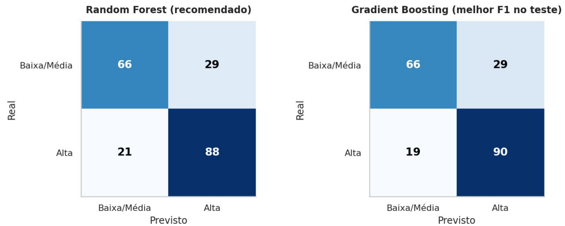
Figura 12 — Matrizes de confusão no conjunto de teste (corte \geq 6 ): recomendado \times melhor F1.
