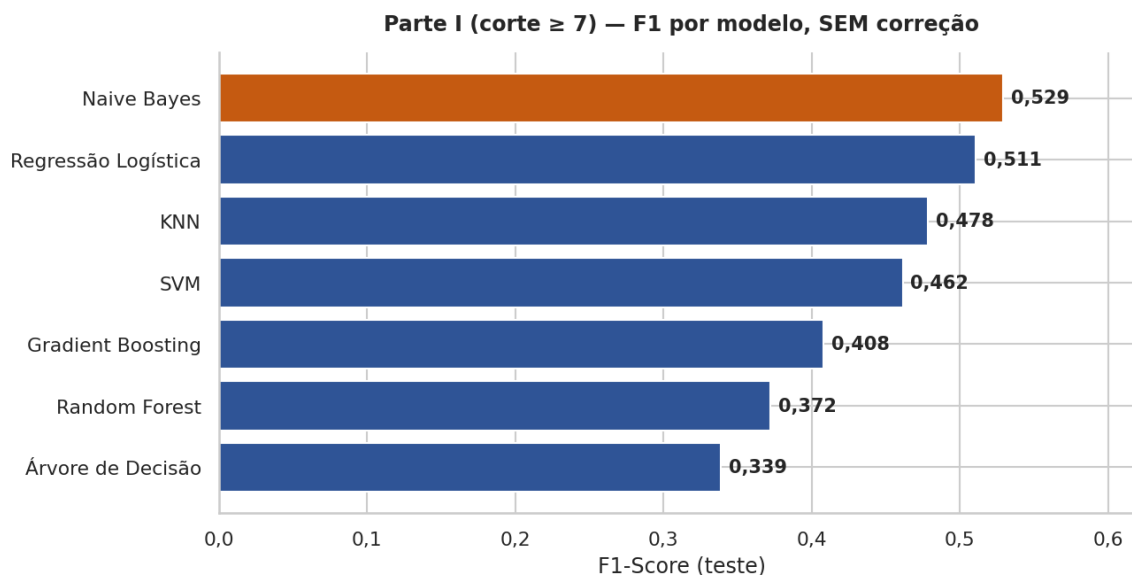
Figura 9 — F1-Score por modelo na Parte I, sem correção (destaque para o melhor).
