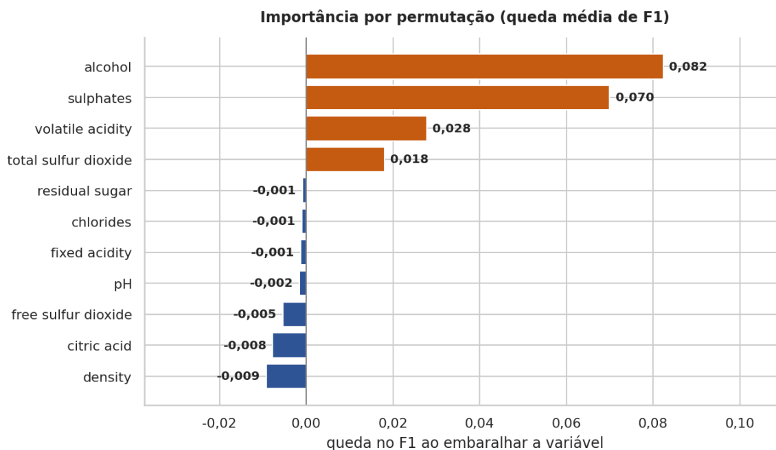
Figura 18 — Importância por permutação (queda média de F1), gráfico revisado.
