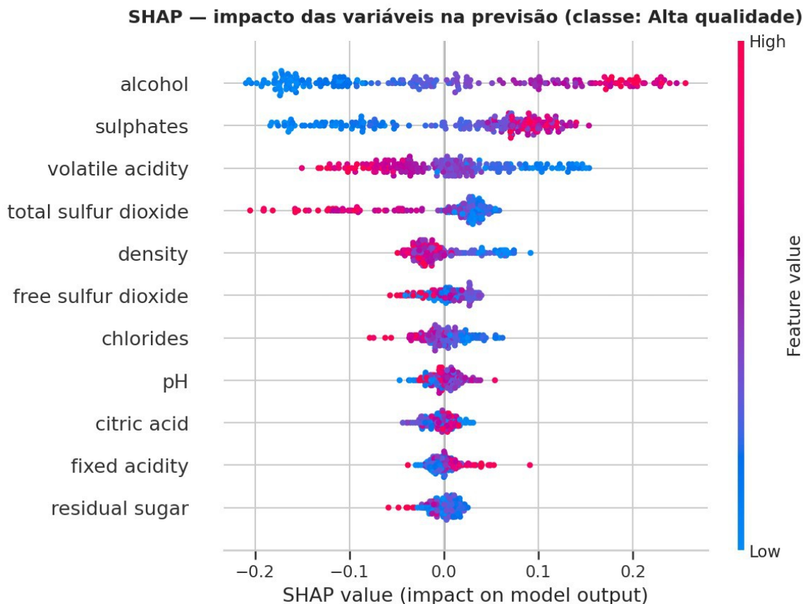
Figura 16 — Resumo SHAP: impacto de cada variável na previsão da classe “Alta qualidade”.
